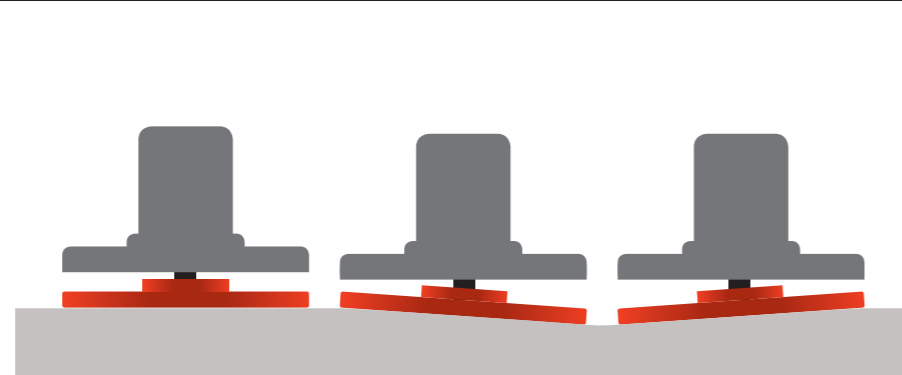
Die Patentierte Kraftübertragung mit kardanischer Aufhängung sorgt für vollflächige Padauflage, vermeidet Beschädigungen und erzeugt ein gleichmäßiges Polierbild
