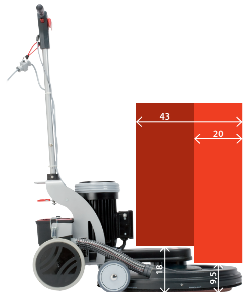
Sehr niedrige Unterfahrhöhe (Angabe in Zentimeter)
