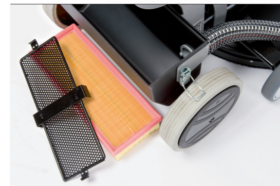
Die integrierte Absaugung nimmt Polierstaub und Abrieb im Filtersystem auf, vorteilhaft in staubsensiblen Umgebungen (z. B. Krankenhäuser)
